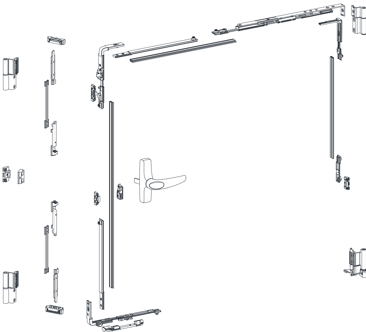
Fig. 5. Schema/esploso dei principali accessori del campione sottoposto a prova
