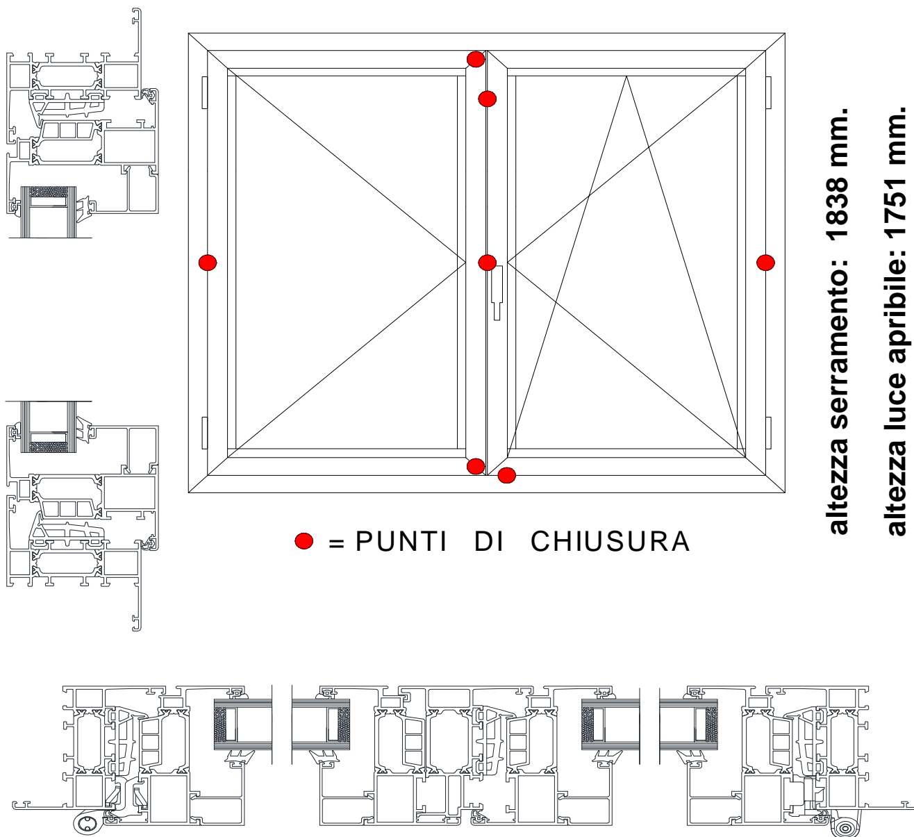
Fig. 1. Prospetto con indicazione dei punti di chiusura e sezioni orizzontale e verticale del campione sottoposto a prova, vista interna
