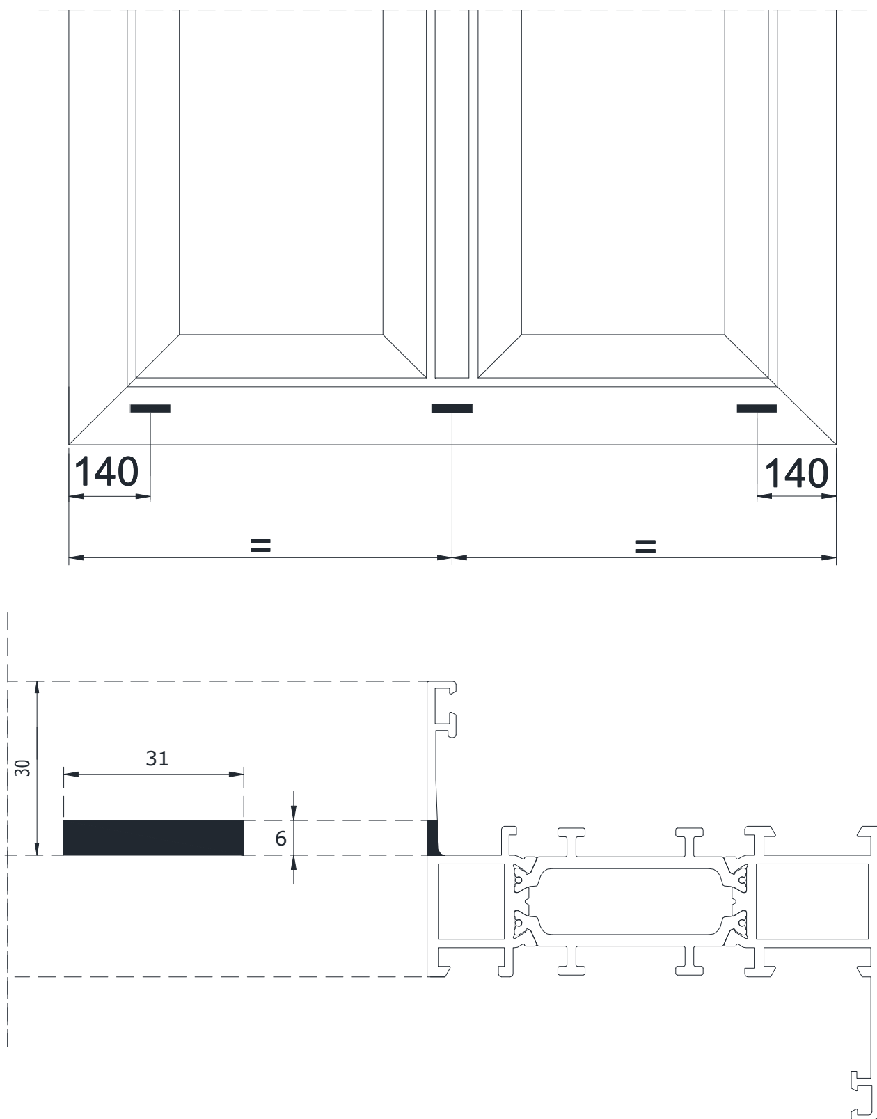
Fig. 4. Dettaglio del sistema di drenaggio del campione sottoposto a prova (dimensioni nominali dichiarate, espresse in mm)
