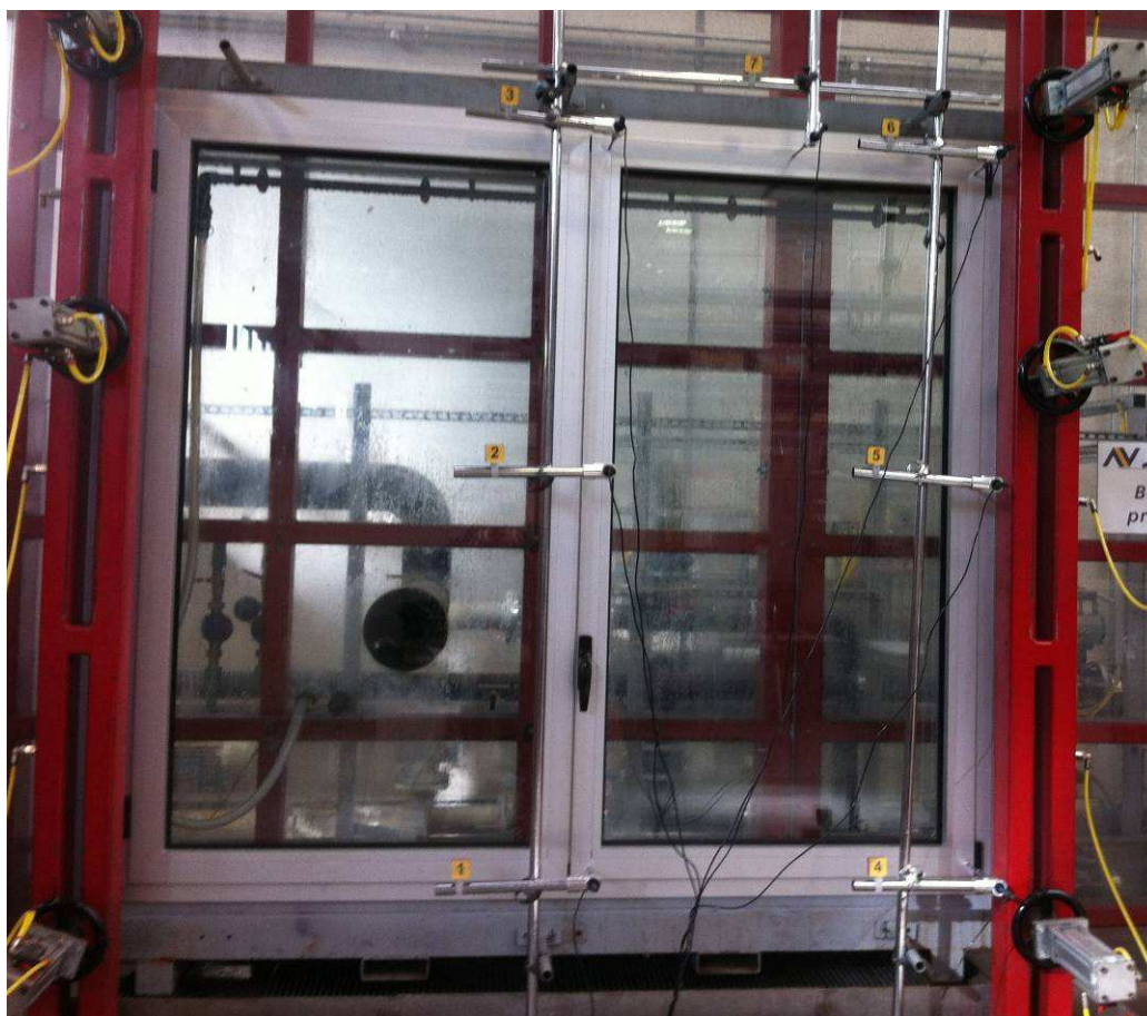
Foto 2. Campione sottoposto a prova durante i test di resistenza al vento (prova di deformazione)
